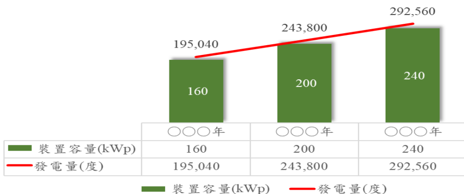
近3年太陽能系統發電量比較
