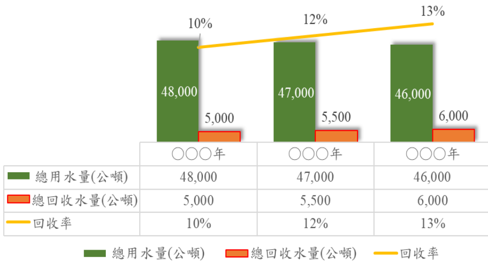
近 3 年製程用水回收率比較
